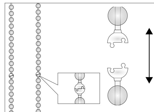
Dispositif de sécurité par ouverture automatique de la chaînette
