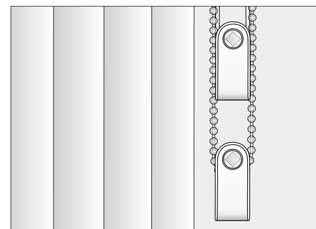
Dispositif de sécurité enfants pour les stores équipés de deux éléments de manoeuvre
